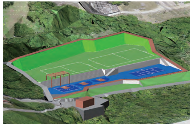
計画(3Dモデル)+現況(オルソ画像)作成イメージ
